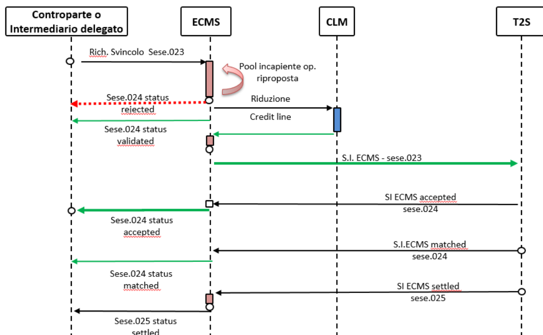
Figura 10 - workflow svincolo A2A
