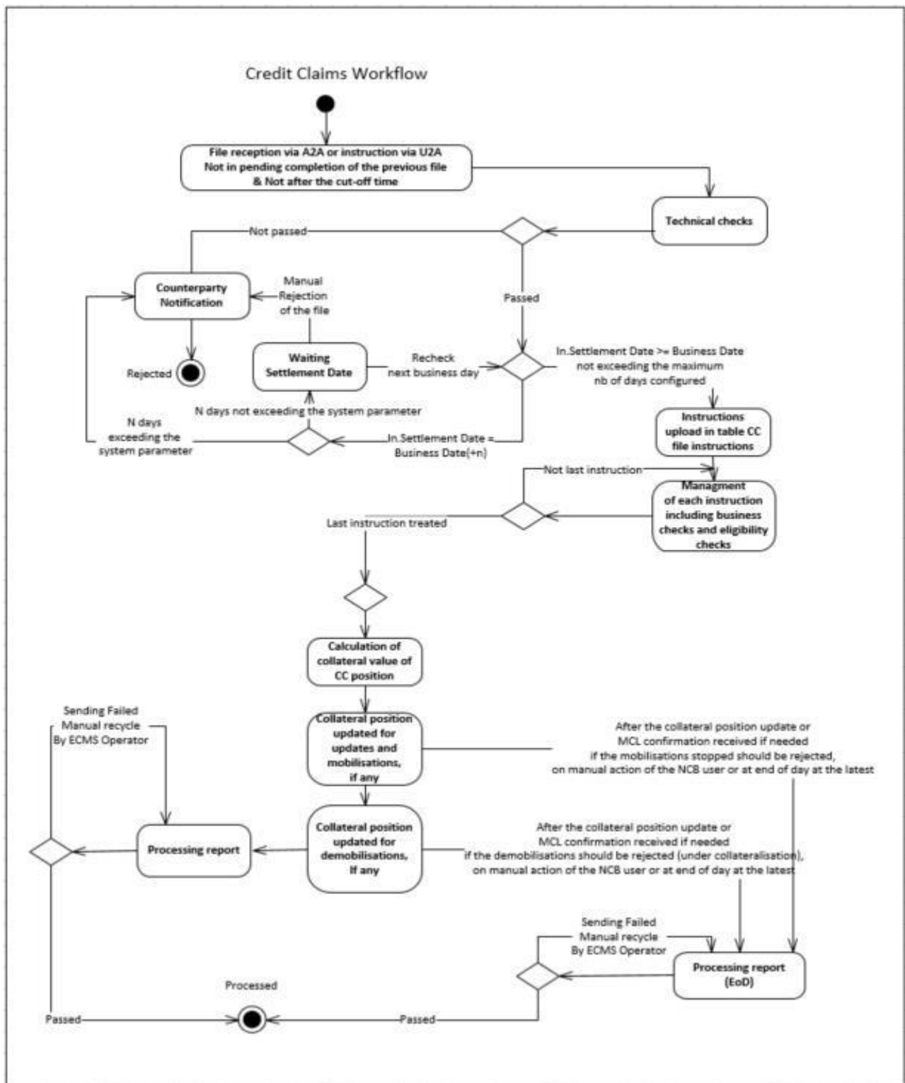
Figura 12 - Flusso di elaborazione di un Credit Claim File
