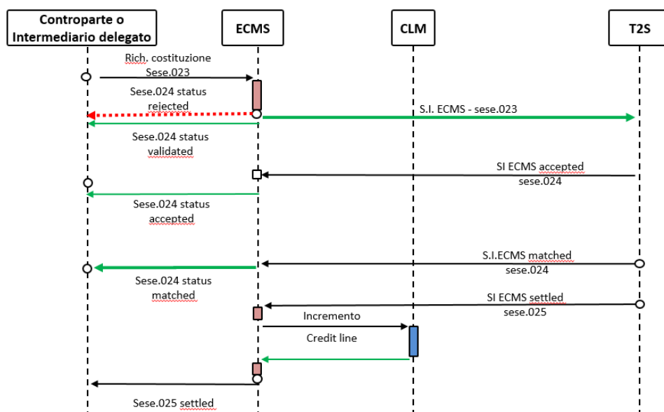
Figura 9 - workflow conferimento A2A
